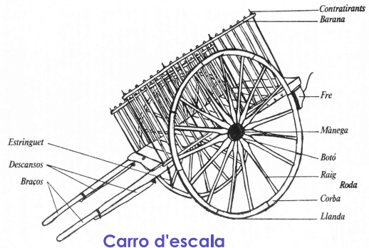
Carro d'escala
